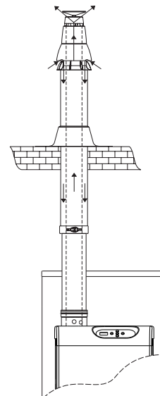
Illustration: Systèmes d'alimentation en air et évacuation des fumées
