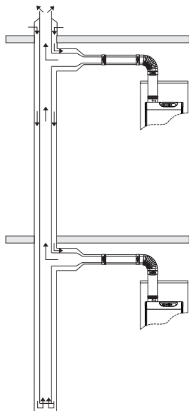
Illustration: Systèmes d'alimentation en air et évacuation des fumées
