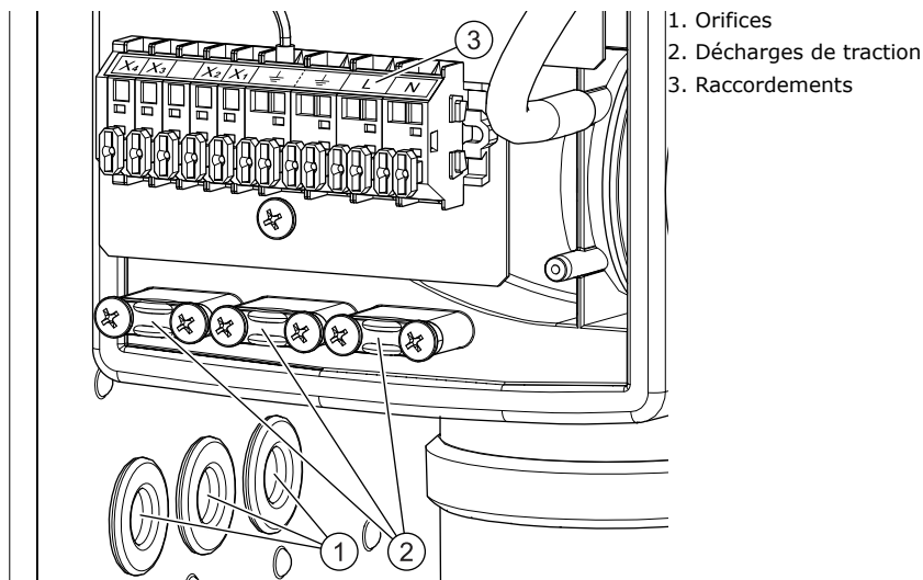
Illustration: Répartiteur
